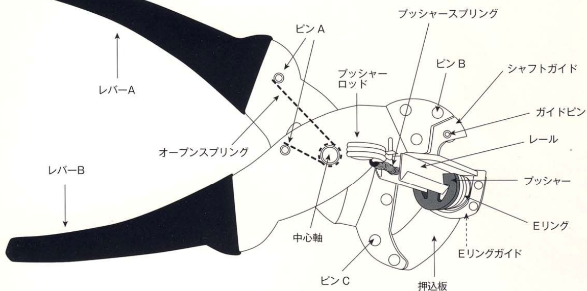
ブッシャー Assy=ブッシャー+ブッシャーロッド+ブッシャースプリング
